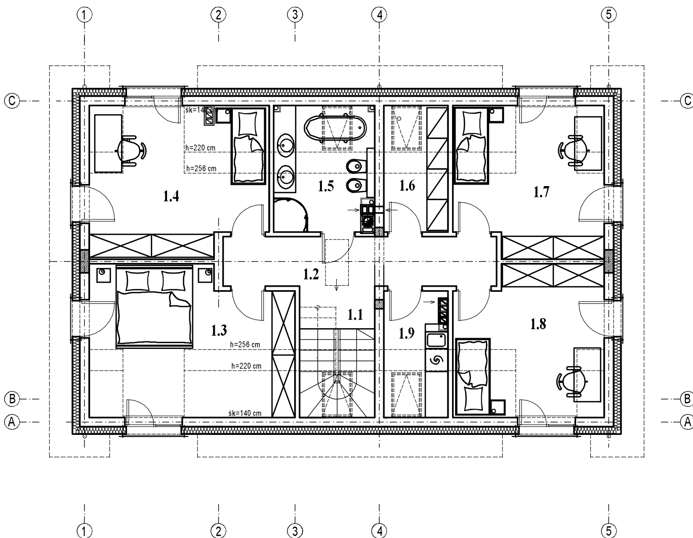
RZUT PODDASZA 1:100
